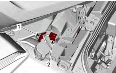
1. B.U.D.S. 的诊断接头 2. OBD2 6 针接头
