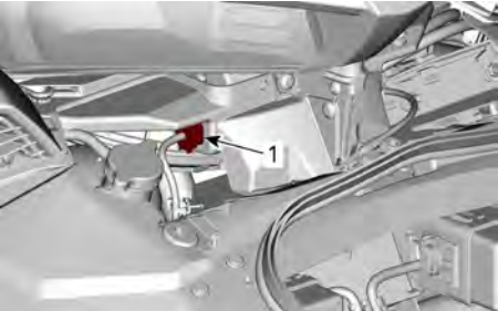
1. B.U.D.S. 的诊断接头
