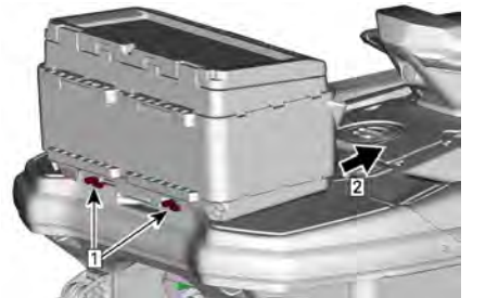
1. 解除冷藏箱的锁定 2. 抬起并向前推
