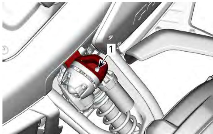
1. Dekselskrue nærlys
