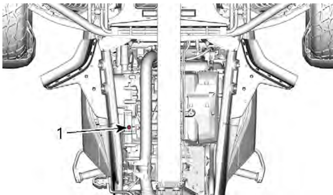
1. Clutchdeksel, magnetisk tappeplugg
