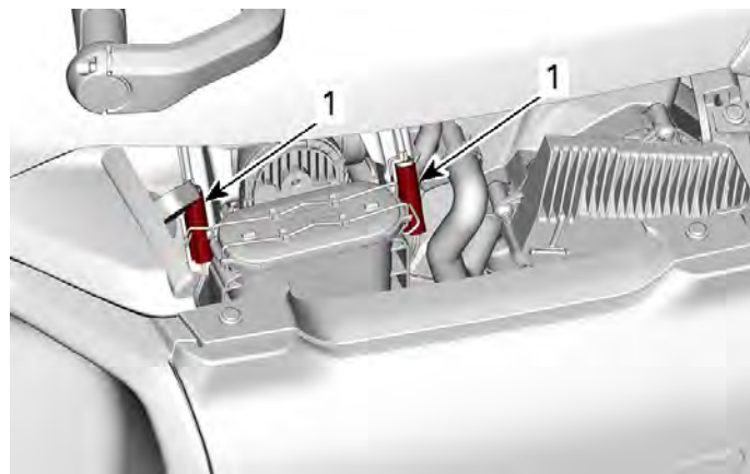
1. Aansluitingen remvloeistofpeilschakelaar
