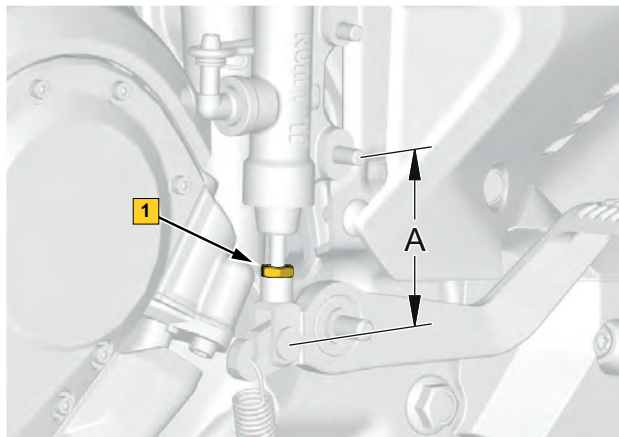
1. Moer hoofdcilindervork
