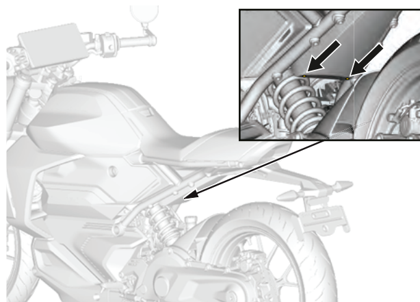
Plaats waterafvoeropeningen
