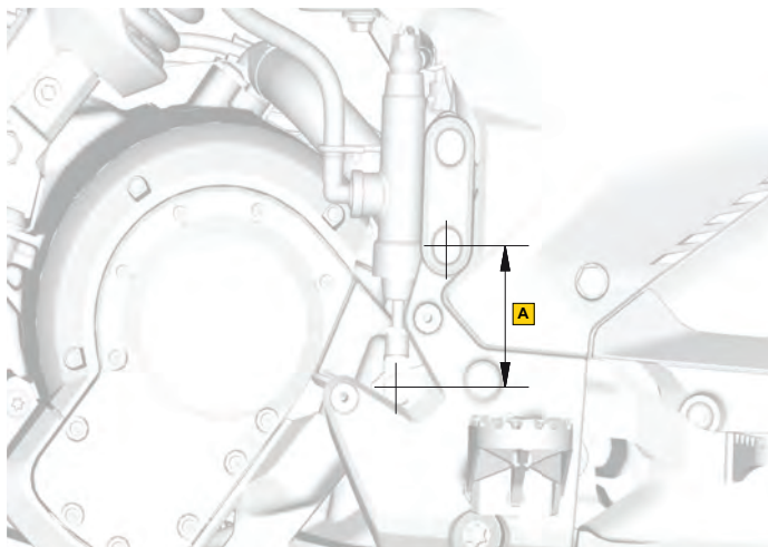
A. Säädön toleranssi 67,5 \pm 3 \text{ mm} ( 2,56 \pm 0,12 \text{ in} )
