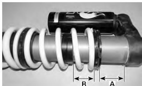
TYPBILD - JUSTERING AV DELNINGS-PUNKT - BAKRE STÖTDÄMPARE
