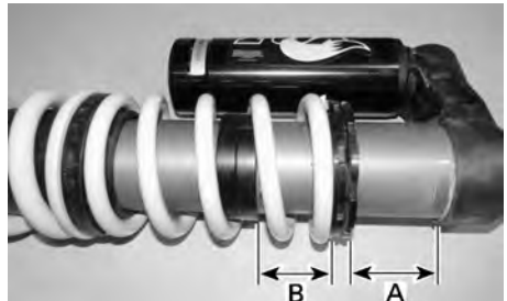
TYPEBILDE – OVERGANGSJUSTERING - STØTDEMPER BAK
