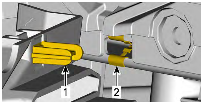
1. Tabulator 2. Klemme
