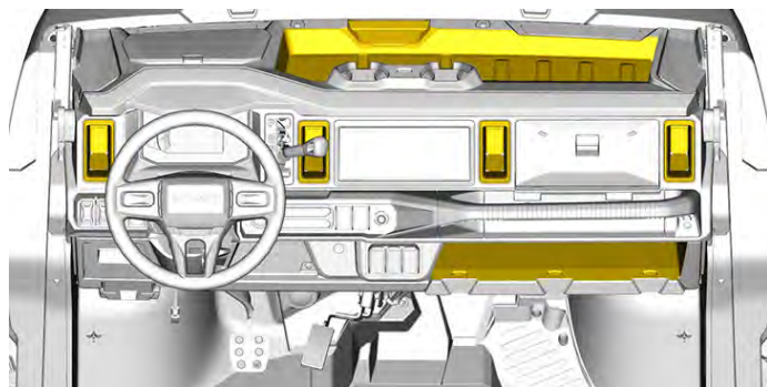
Modellen zonder HVAC
