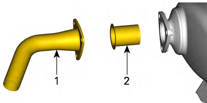
1. Utblåsningsrør 2. Gnistfanger
