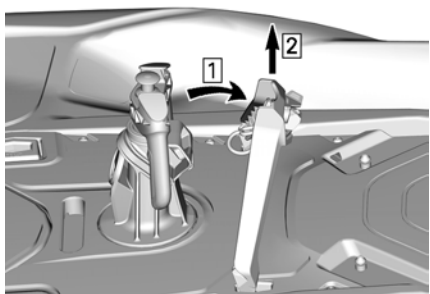
1. Kippträger 2. Hebeträger
