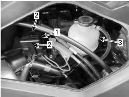
1. Cubierta de la caja de fusibles 2. Pestañas de bloqueo 3. Depósito de expansión
