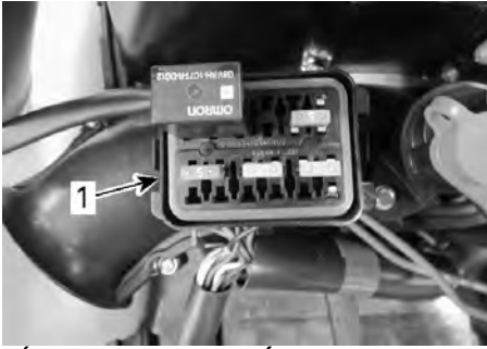
TÍPICO - TAPA EXTRAÍDA DE LA CAJA DE FUSIBLES
