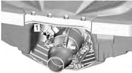
1. Anschluss des Strahlpumpenträgers
