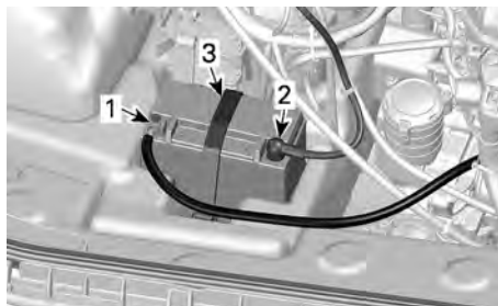
MITTLERE KAROSSERIE AUS GRÜNDEN DER ÜBERSICHTLICHKEIT ENTFERNT
