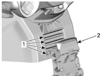
TYPISCH – VERRIEGELUNG DER LENKSÄULENVERSTELLUNG GESICHERT
