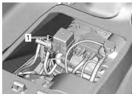
1. Scatola fusibili
