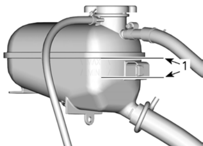
KOELVLOEISTOFEXPANSIEVAT
