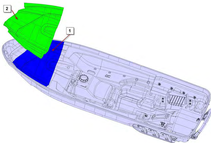
POSIÇÃO DA CAMADA DE REFORÇO 1 E 2
