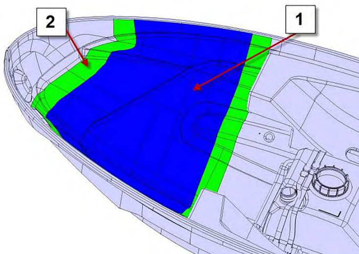
POSIÇÃO DA CAMADA DE REFORÇO 1 E 2
