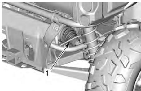
1. Indre drivakselmansjetter
