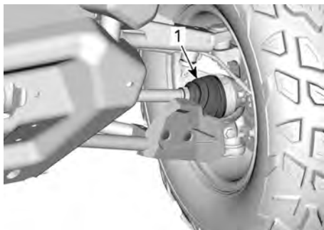
1. Ytre drivakselmansjetter
