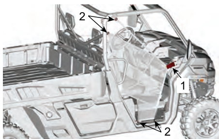
CÔTÉ PASSAGER
