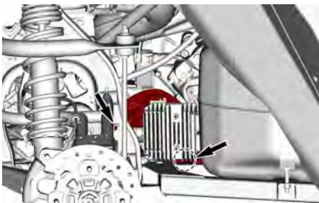
EMPLACEMENT DES FIXATIONS DU SUPPORT DU RÉGULATEUR DE TENSION
