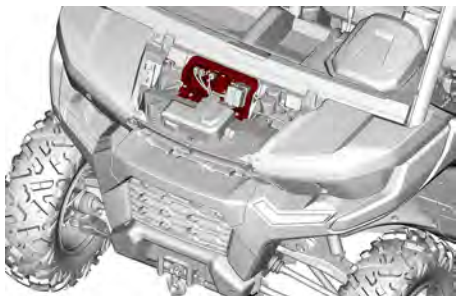
保险丝盒支架
