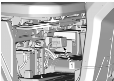
1. 后部辅助保险丝盒
