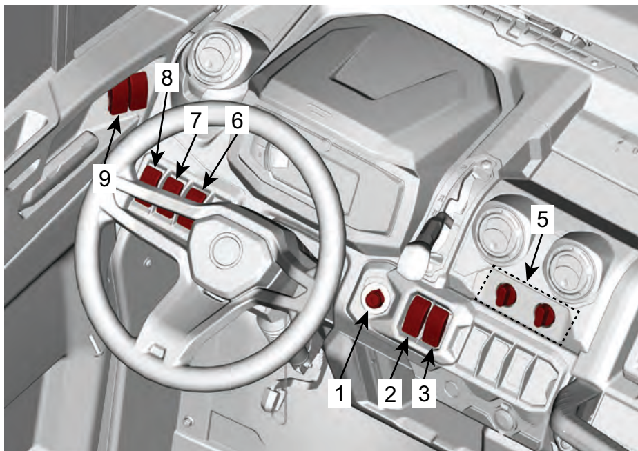
TÍPICO: MODELO CON CABINA CON SISTEMA DE CALEFACCIÓN MOSTRADO
