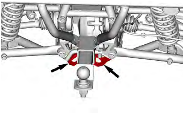
Hintere Abschlepphaken
