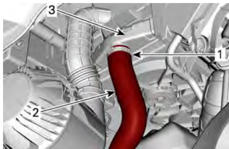
LINKER ACHTERWIELKUIP
