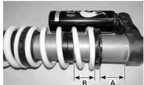
SITUAZIONE TIPICA - REGOLAZIONE CROSSOVER - AMMORTIZZATORE POSTERIORE
