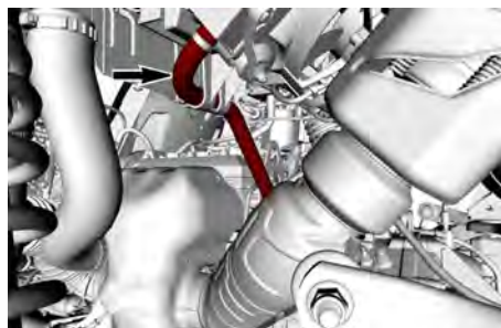
TUBO FLESSIBILE INFERIORE DEL RADIATORE – VANO RUOTA POSTERIORE SINISTRO
