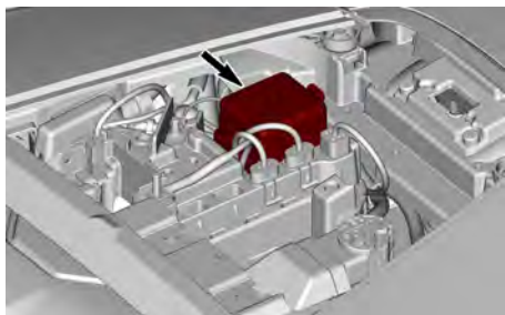
SCATOLA FUSIBILI ANTERIORE
