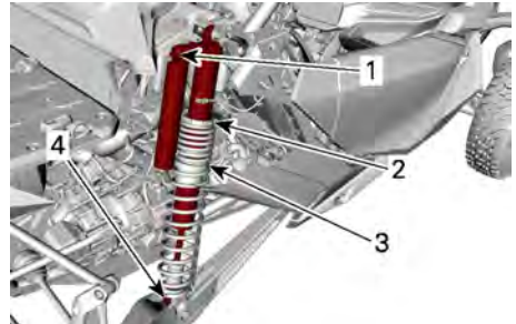
TIPIQUE - SUSPENSION ARRIÈRE
