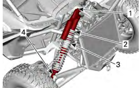
TIPIQUE - SUSPENSION AVANT
