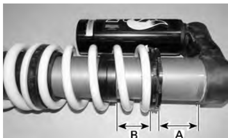
TÍPICO - AJUSTE DE LA SUPERPOSICIÓN - AMORTIGUADOR TRASERO
