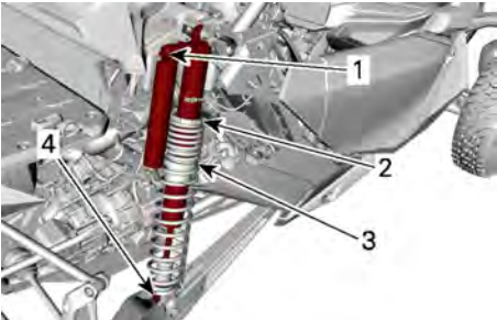
TÍPICO - SUSPENSIÓN TRASERA
