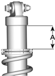
A = DISTANCE DE RESSORT PRÉCHARGÉ
