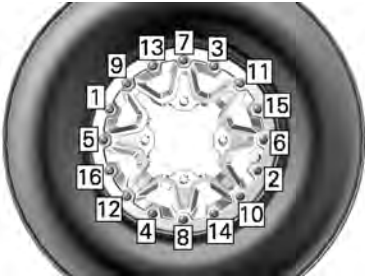
典型示例 - 紧固顺序
