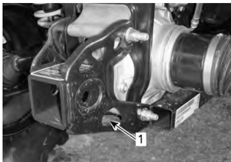
1. 后栓系点的位置
