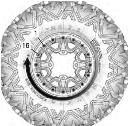
典型示例 - 最终紧固顺序
