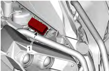
1. 主保险丝支座
