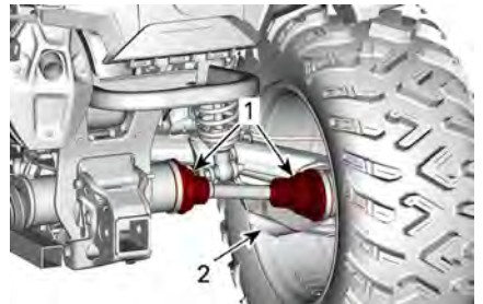
TYPEBILDE – BAK PÅ KJØRETØYET
