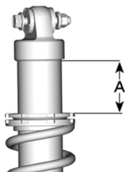
A = AVSTAND FOR FORHÅNDSBELASTNING AV FJÆREN
