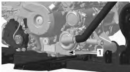
1. Koelvloeistofaftapplug
