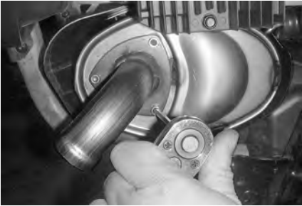
TÍPICO - RETIRE EL TUBO DE ESCAPE.
