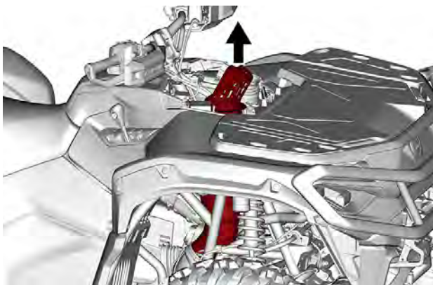
5. Fjern klemmeskruen på spoleledningen.
