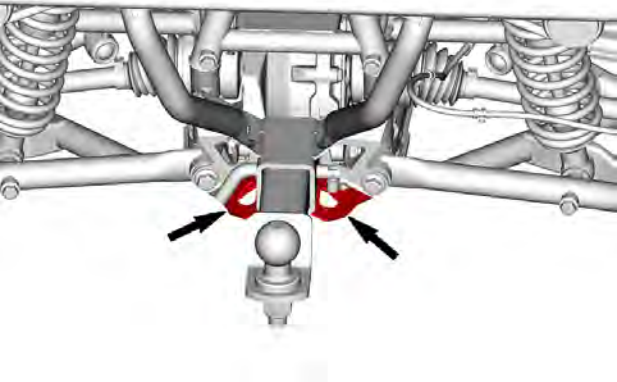
Sleephaken achter
