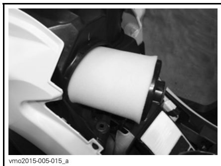
BORTTAGNING AV LUFTFILTER
