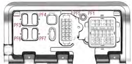
STEUN ZEKERINGDOOS
