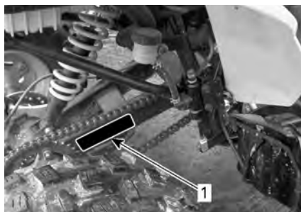
1. Posizione etichetta regolazione catena di trasmissione
