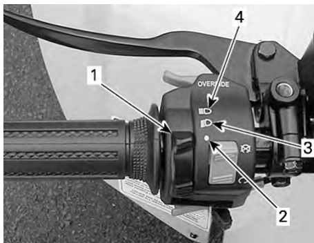
SITUAZIONE TIPICA — FUNZIONI DELL'INTERRUTTORE DEL FARO
