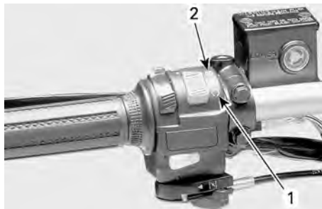
CONFIGURAZIONE TIPICA - INTERRUITTORE DI EMERGENZA PER ARRESTO MOTORE
