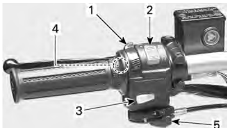
CONFIGURAZIONE TIPICA — INTERRUITTORE MULTIFUNZIONE
