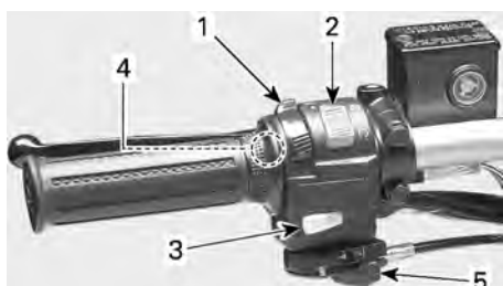
TYPIQUE - MULTIFONCTION
