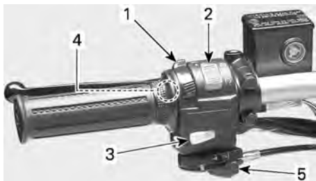
TYPISCH MULTIFUNKTIONSSCHALTER
