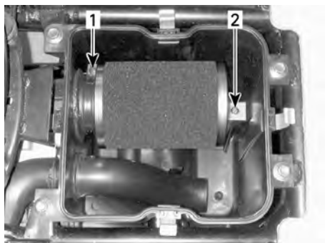
1. Schlauchschelle
