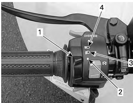
TYPISCH — SCHEINWERFERSCHALTER-FUNKTION
