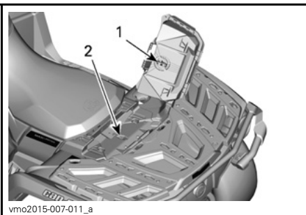
1. Hanskeromlås 2. LINQ-åpning
