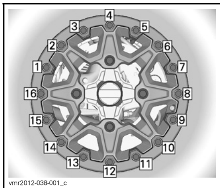
SISTE TILTREKKINGSREKKEFØLGE
