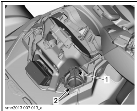
1. CVT-luftfilter 2. Tapp
