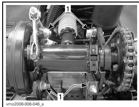
TYPIQUE - ARBRE D'ENTRAÎNEMENT
