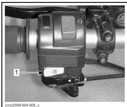
ÉTRANGLEUR OUVERT
