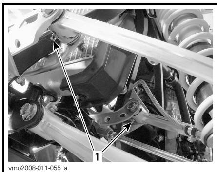
TYPIQUE BRAS DE SUSPENSION SUPÉRIEUR (DS 450 X xc)
