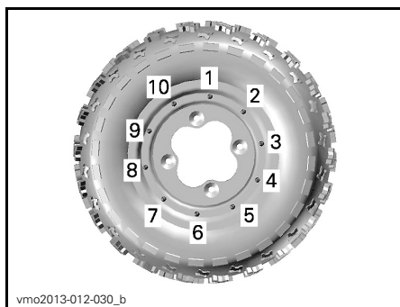
ROUE À VERROU DE TALON À 10 BOULONS — SÉQUENCE DE SERRAGE DE LA DERNIÈRE ÉTAPE
