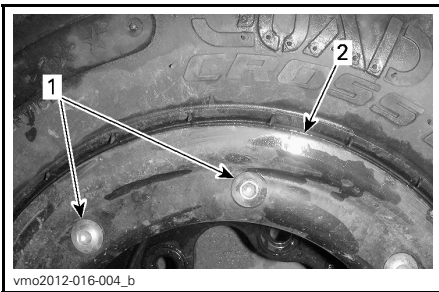
1. Écrous du verrou de talon 2. Anneau de retenue du verrou de talon
