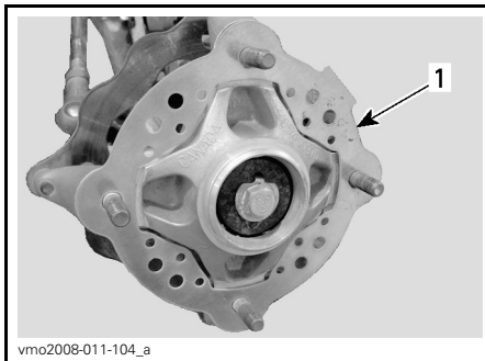
ROUE AVANT
