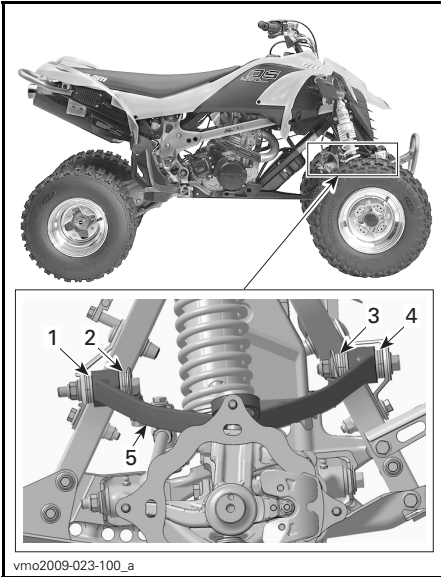
vm02009-023-100_a TYPIQUE POSITION DROITE DES CALES
