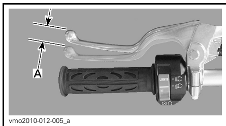
MANETTE D'EMBRAYAGE — JEU LIBRE NOMINAL
