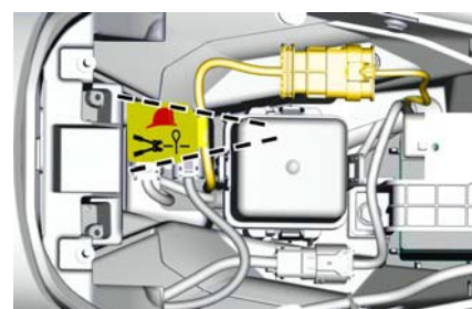
Boucle à couper pour premiers répondants sous le siège
