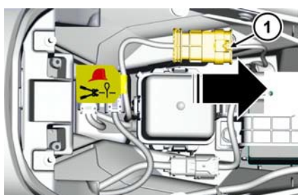
Déconnexion Connecteur sous le siège du conducteur
