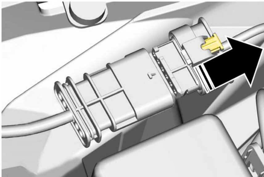
Kuljettajan istuimen alla sijaitsevan FRCL-liittimen irtikytkentä
