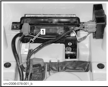
1. Porte-fusibles
