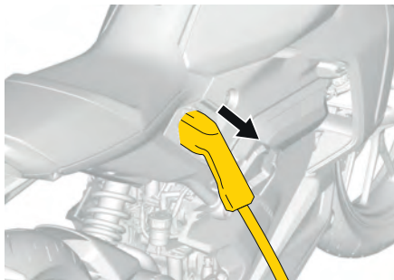
Tyyppin 2 latauskaapelin liitin ( IEC 62196)
