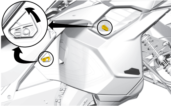
Tyypillinen – 2 salpaa
