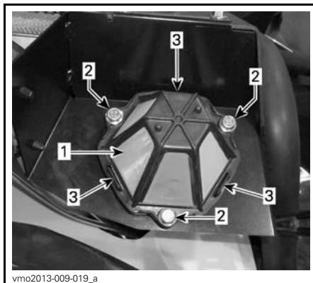
1. Filtre à air de la transmission CVC
